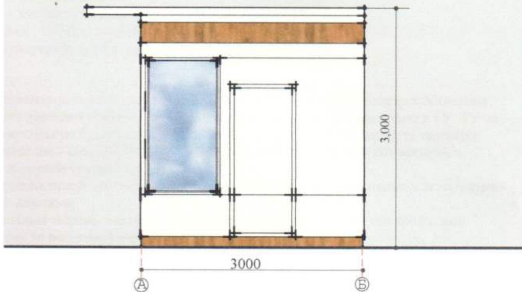
Боковий фасад
