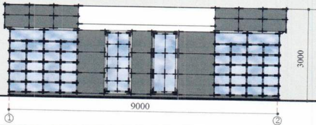
Боковий фасад м. 1:50
