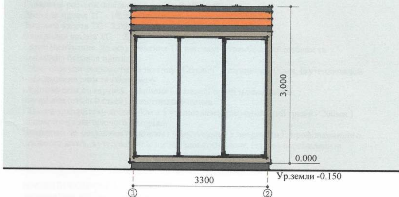
Боковий фасад
