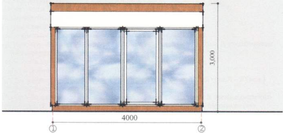
Боковий фасад
