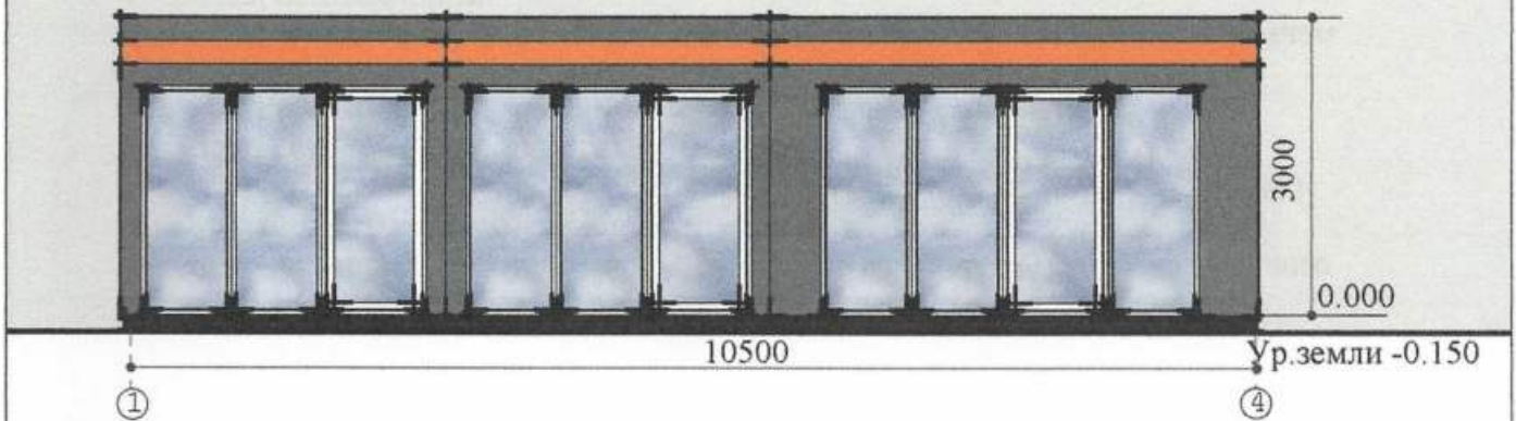
Боковий фасад
