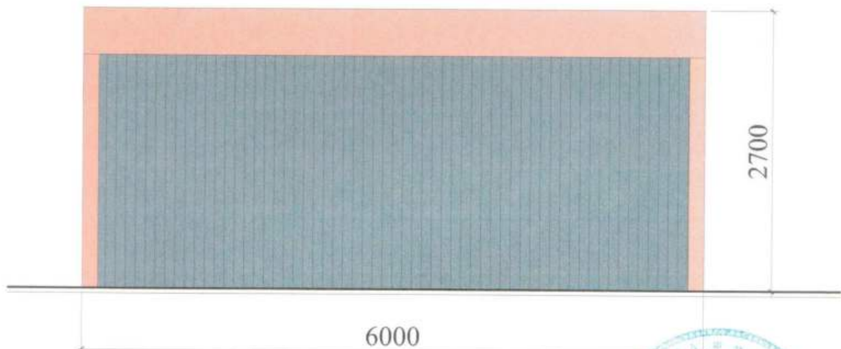
Бічний фасад М 1:50
