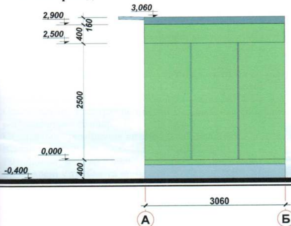
Бічний фасад
