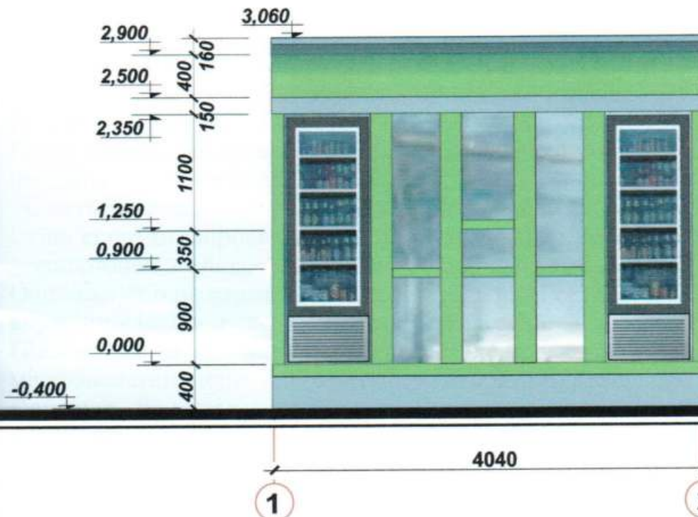
Бічний фасад
