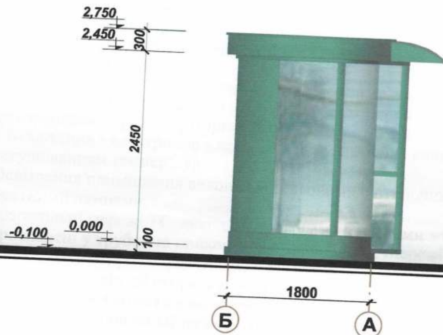
Бічний фасад
