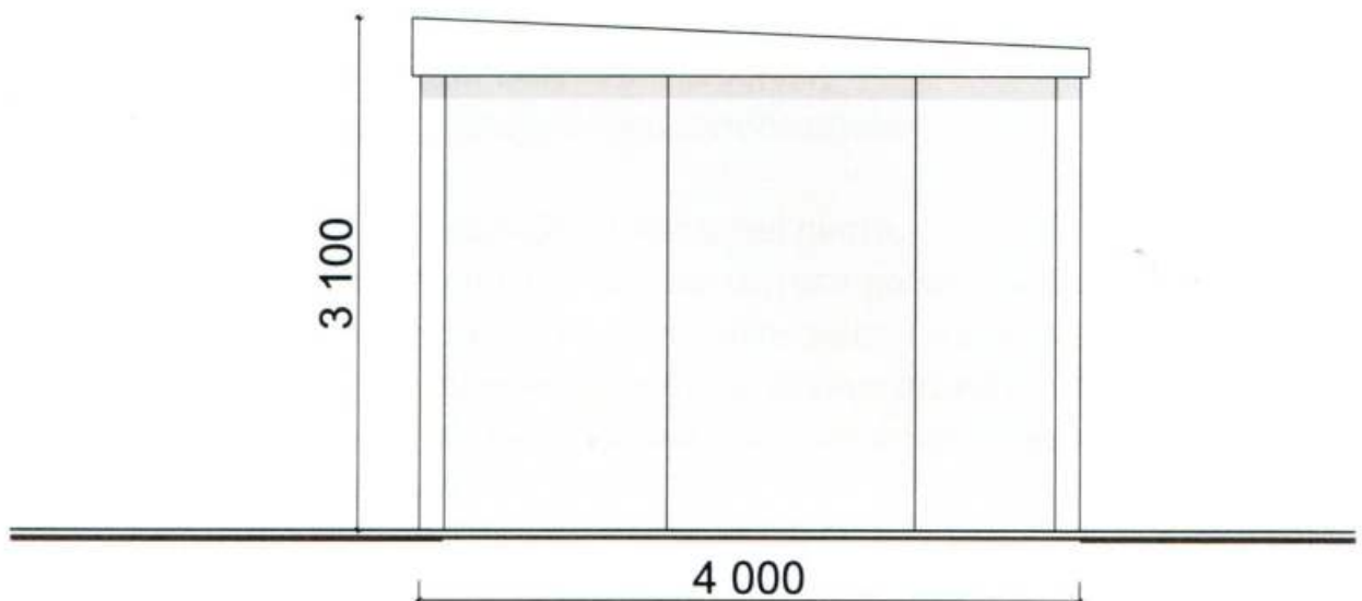
Бічний фасад
