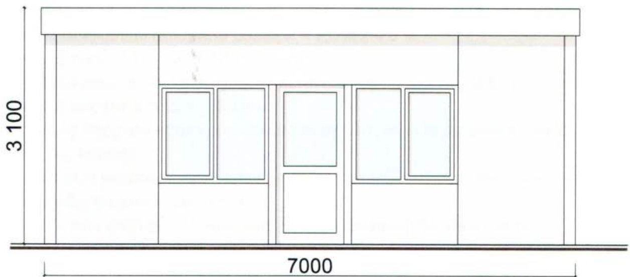
Головний фасад
