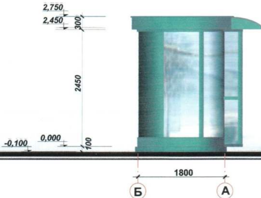
Бічний фасад
