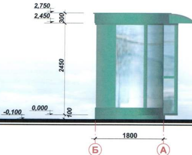
Бічний фасад
