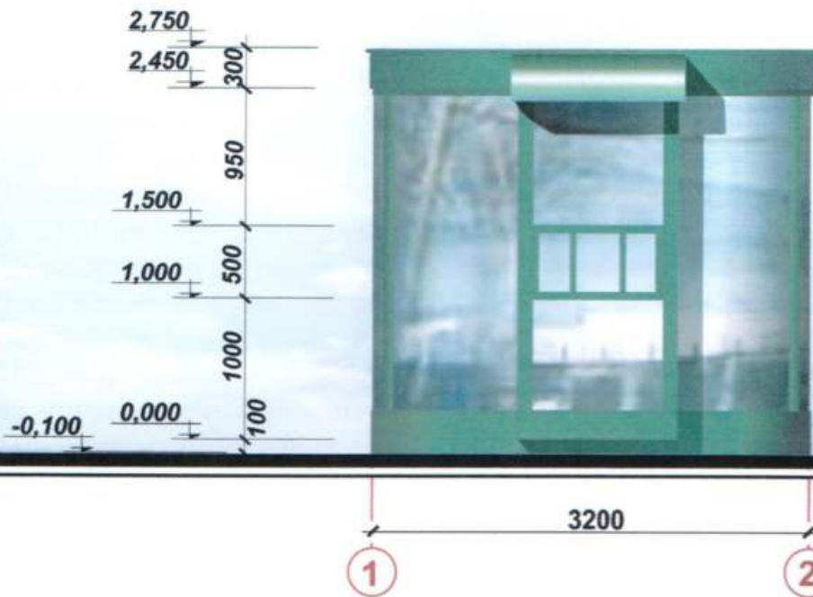
Бічний фасад
