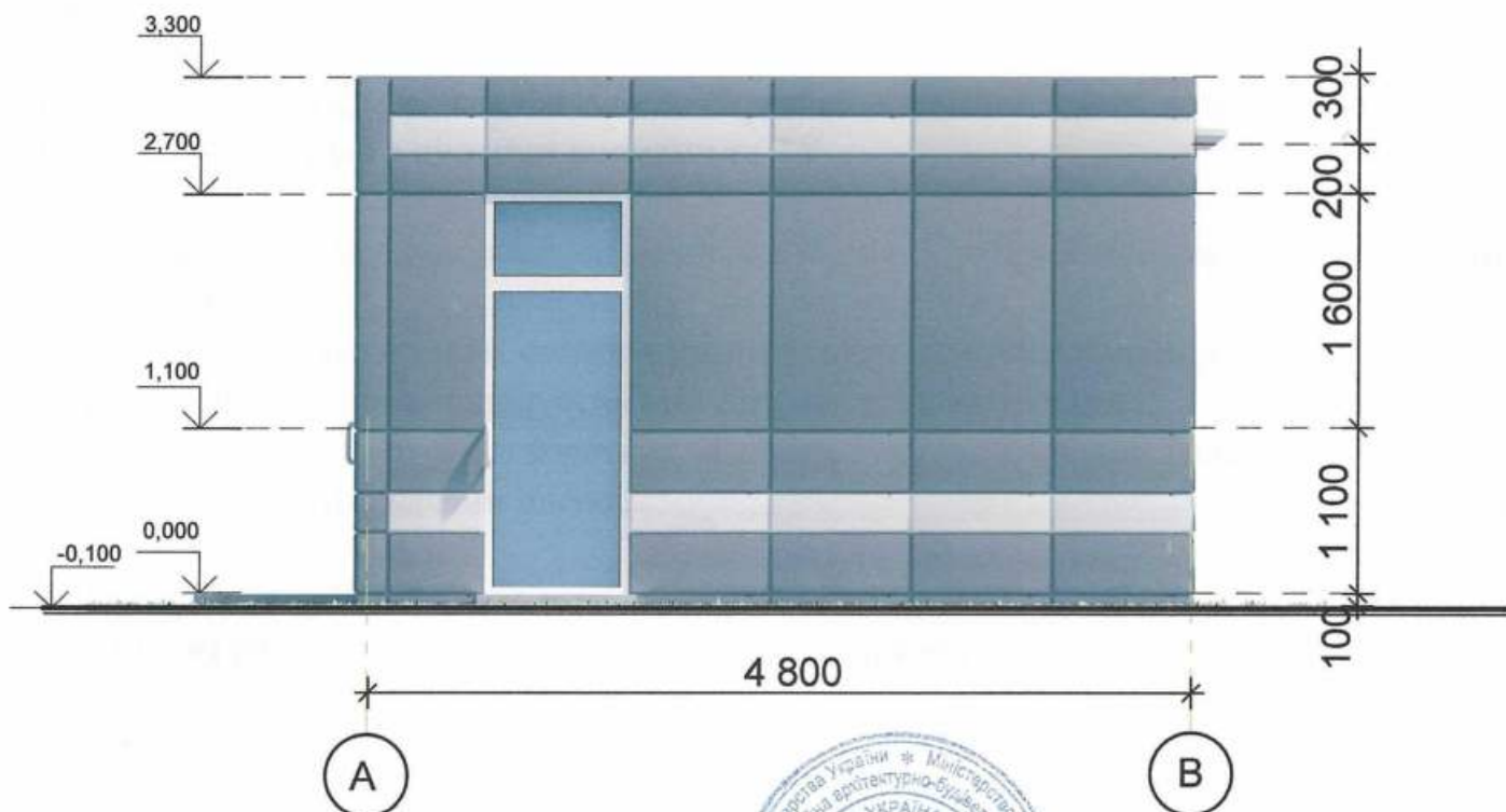
Боковий фасад М 1:50 .
