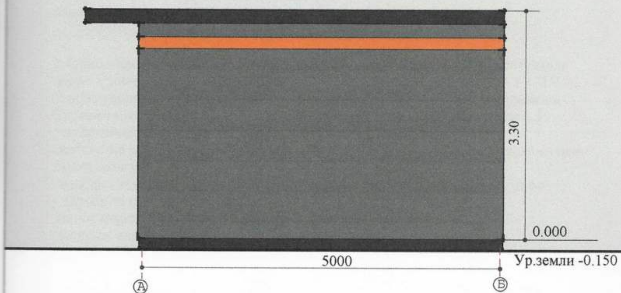
Боковий фасад
