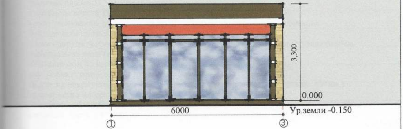
Боковий фасад
