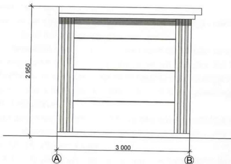
Бічний фасад
