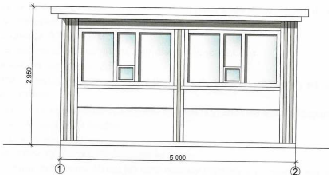
Головний фасад
