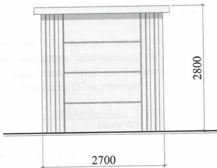
Бічний фасад ТС М 1:50
