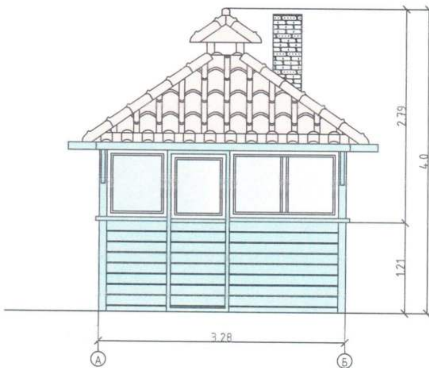
Бічний фасад ТС М 1:50
