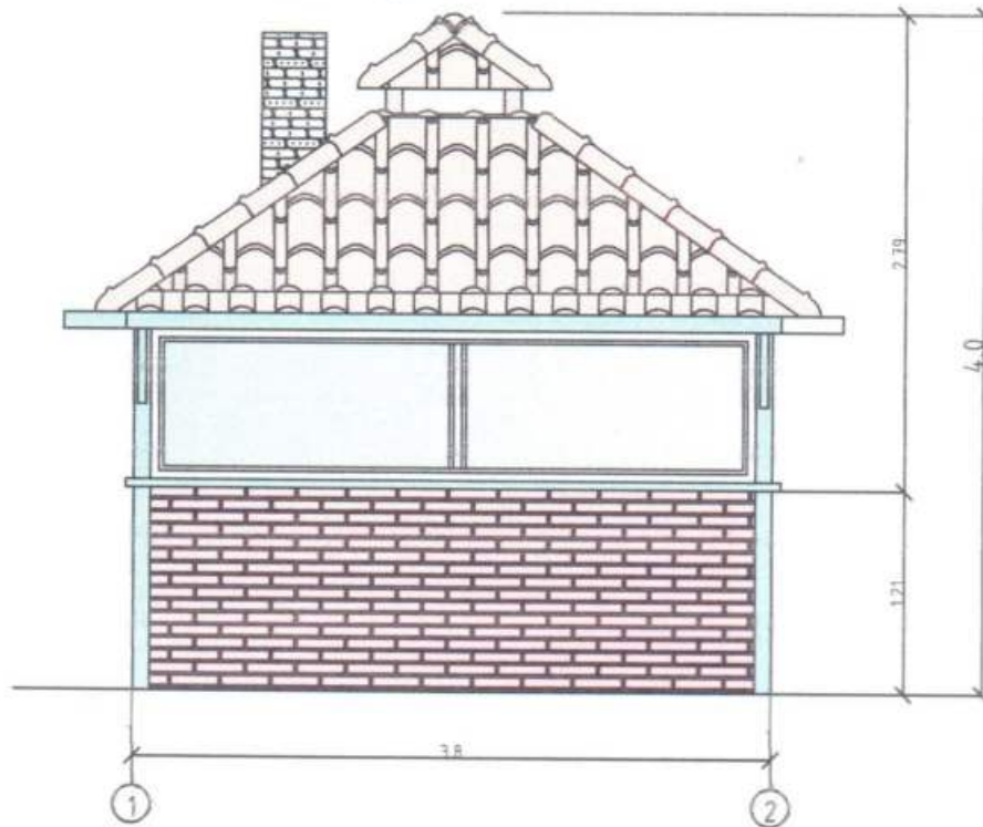
Ескізи фасадів ТС Головний фасад ТС М 1:50
