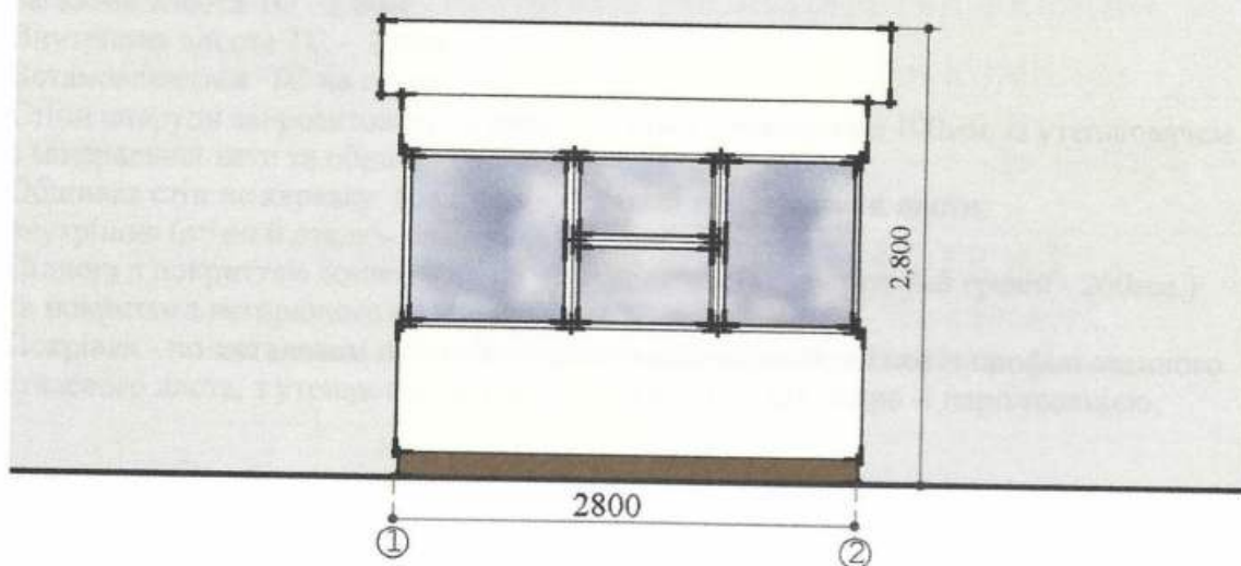
Боковий фасад
