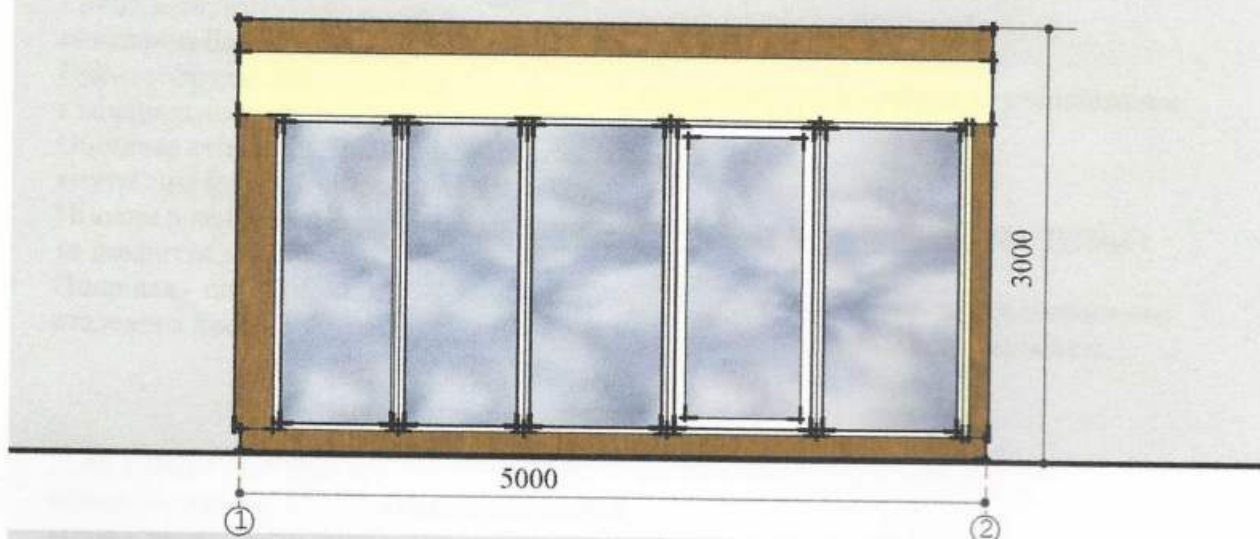
Боковий фасад
