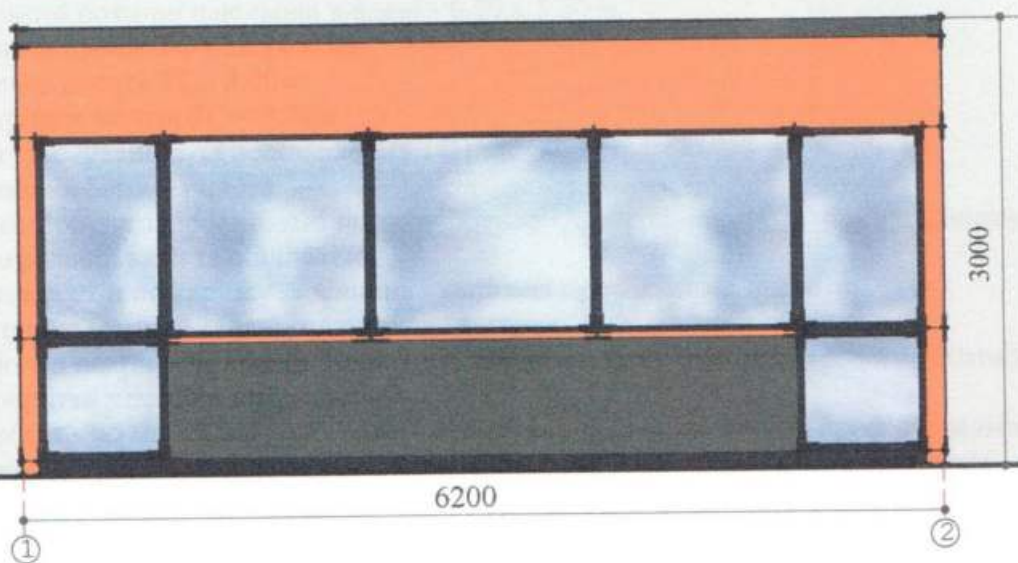
Боковий фасад
