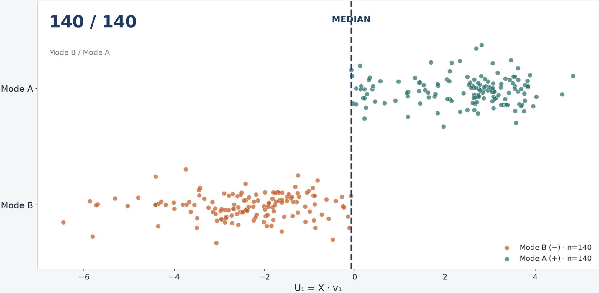
280 МО вдоль главной коллективной оси
