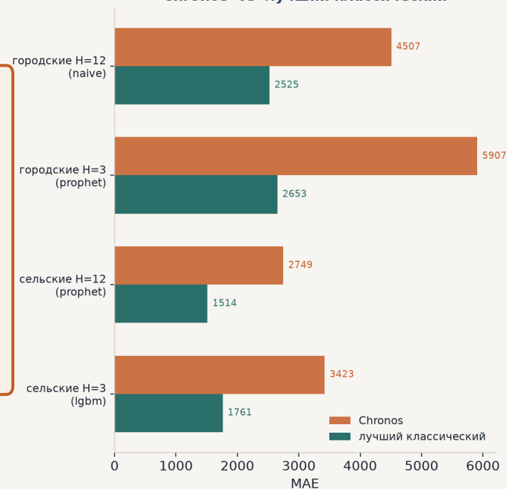
Chronos vs лучший классический
