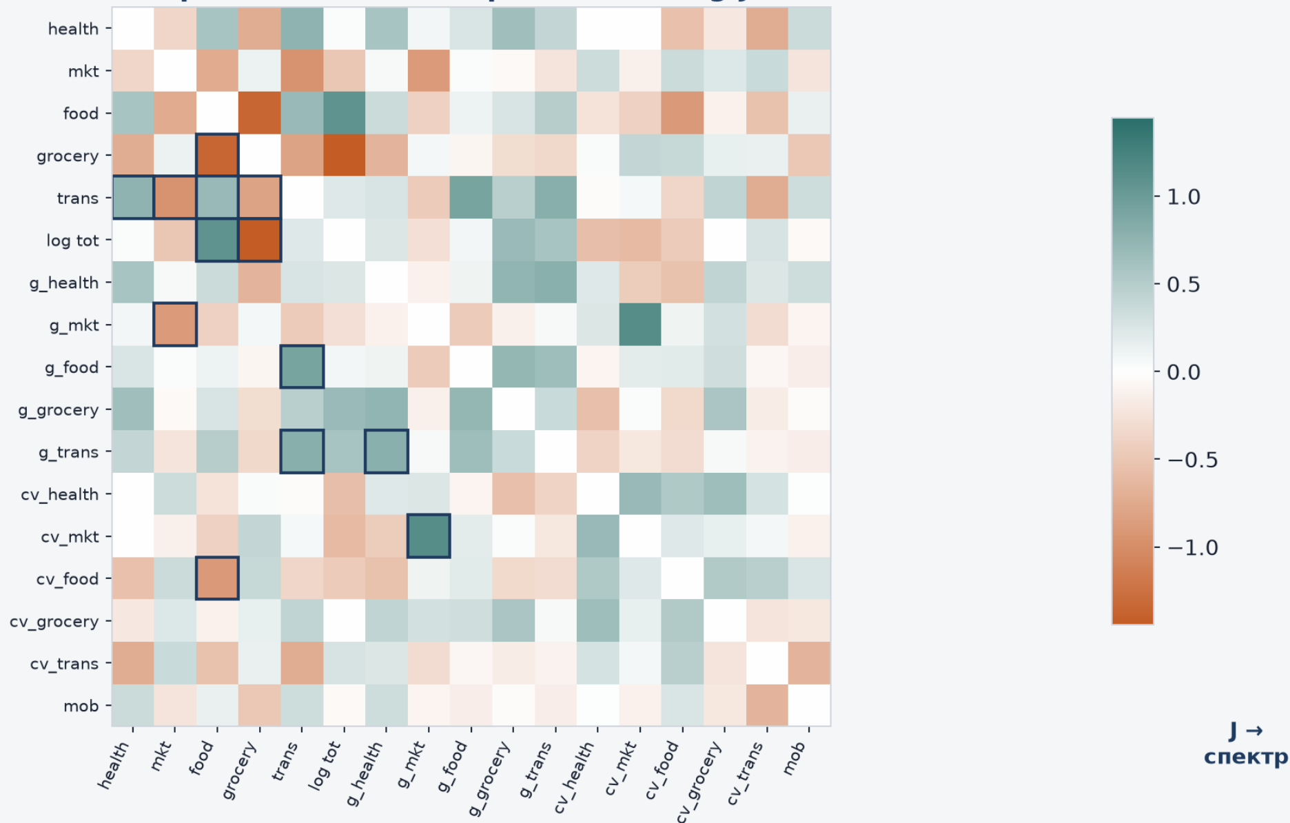
Карта зависимостей признаков · \text{diag}(J)=0
