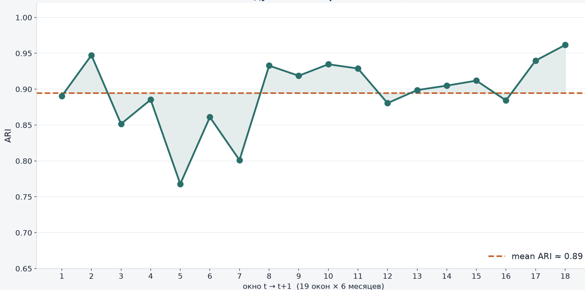
Устойчивость между окнами · перебежчики 49/277 = 17.7%
