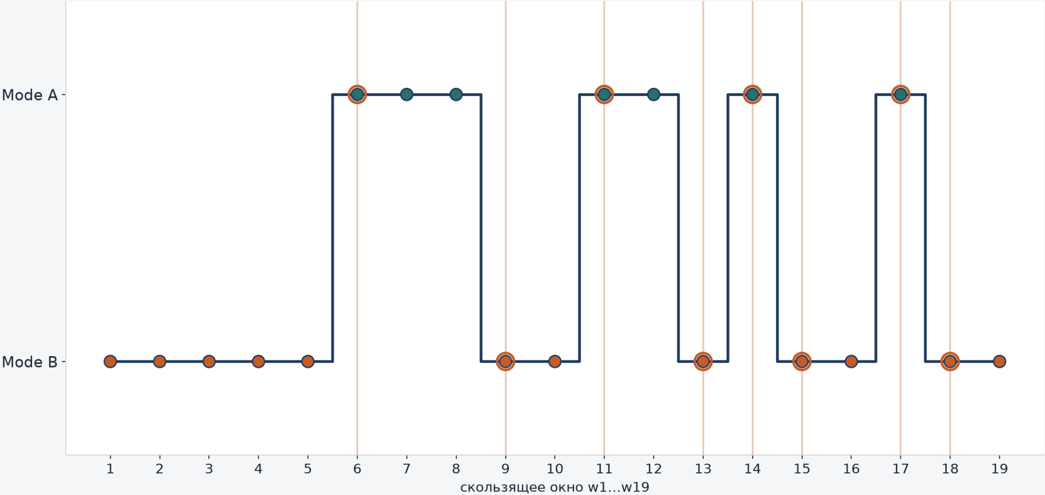
вологодский · 8 переключений / 19 окон
