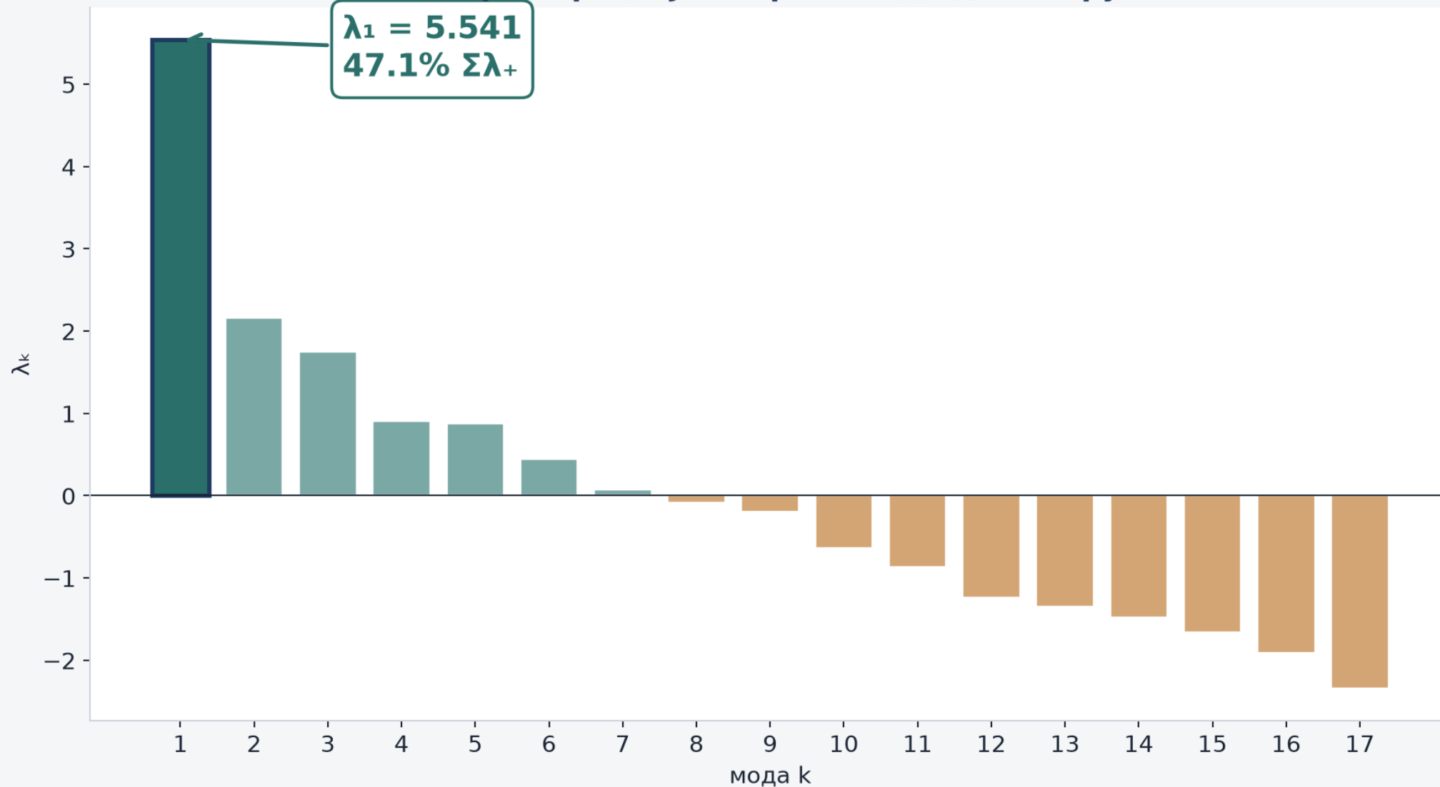
Спектр матрицы J — первая мода доминирует
