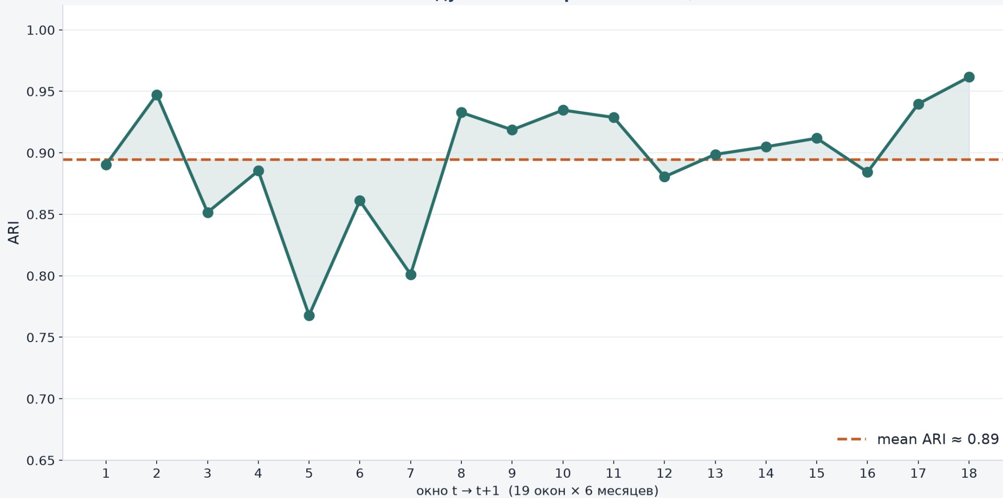
Устойчивость между окнами · перебежчики 49/277 = 17.7%
