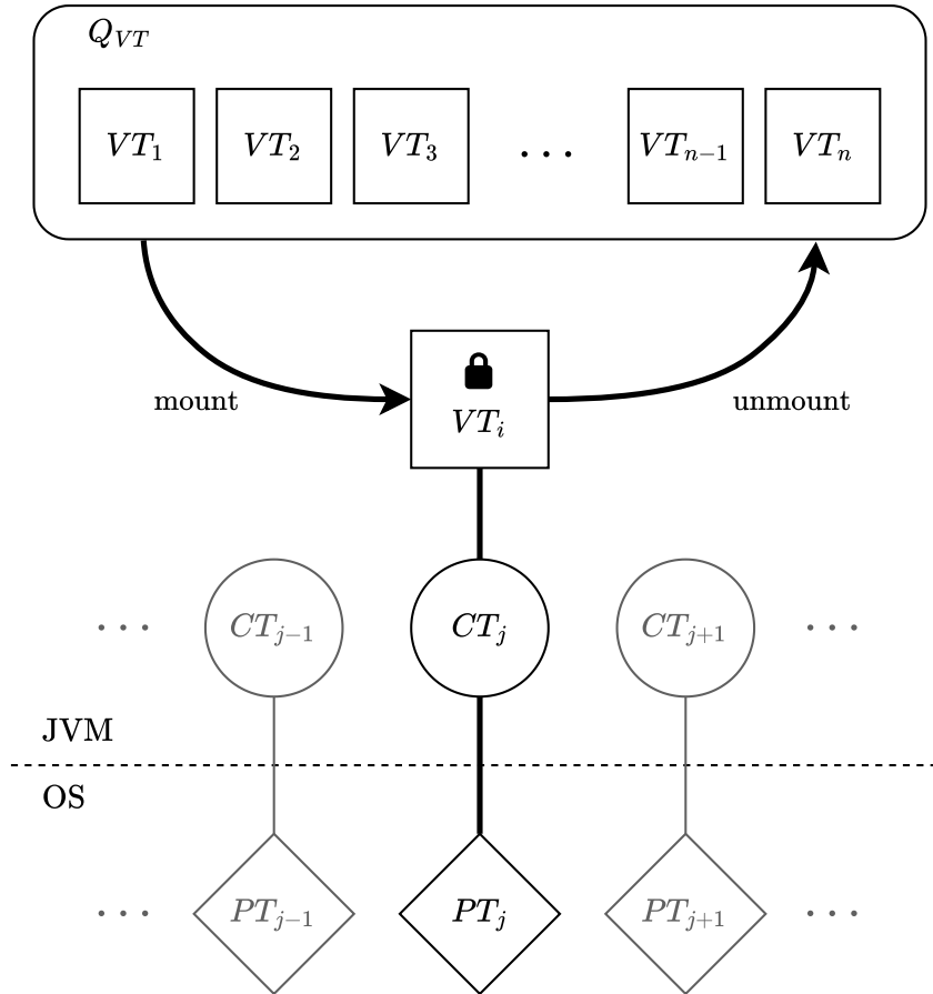
Rysunek 3.1: Cykl życia wirtualnych wątków w środowisku JVM (źródło: opracowanie własne na podstawie [11])
