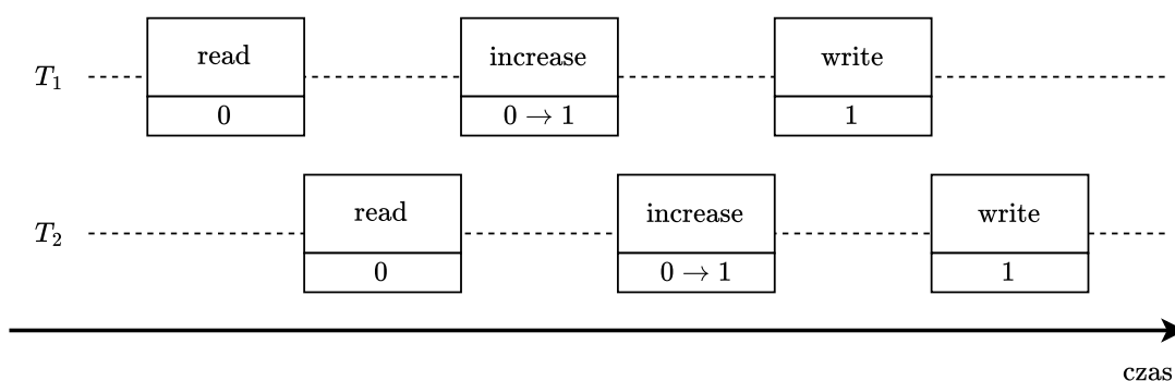
Rysunek 2.2: Ilustracja zjawiska race condition na podstawie wywołania procedury increaseByOne
