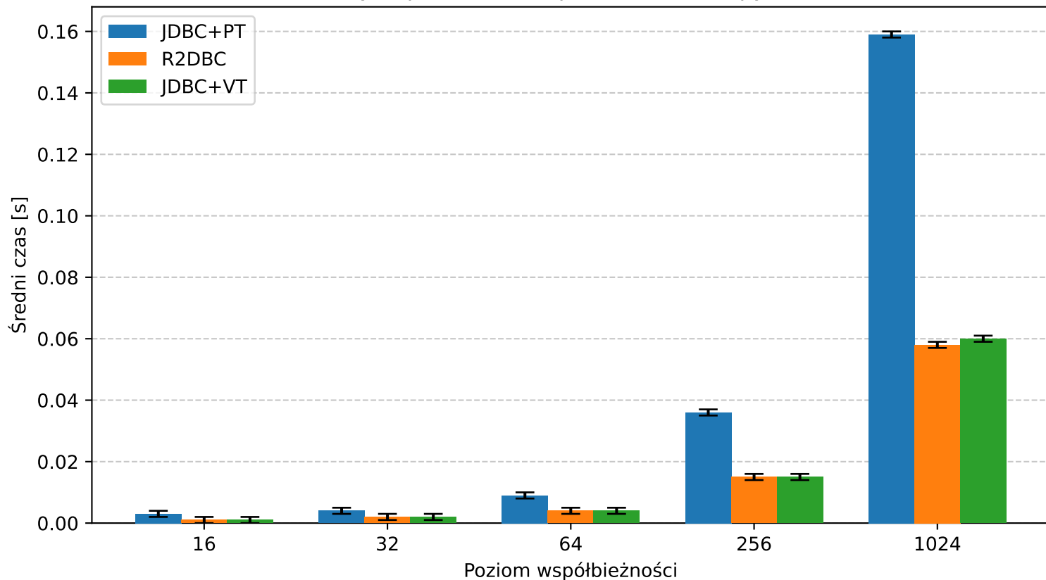
Porównanie średniego czasu trwania operacji dla różnych poziomów współbieżności (zapytanie Q1)
