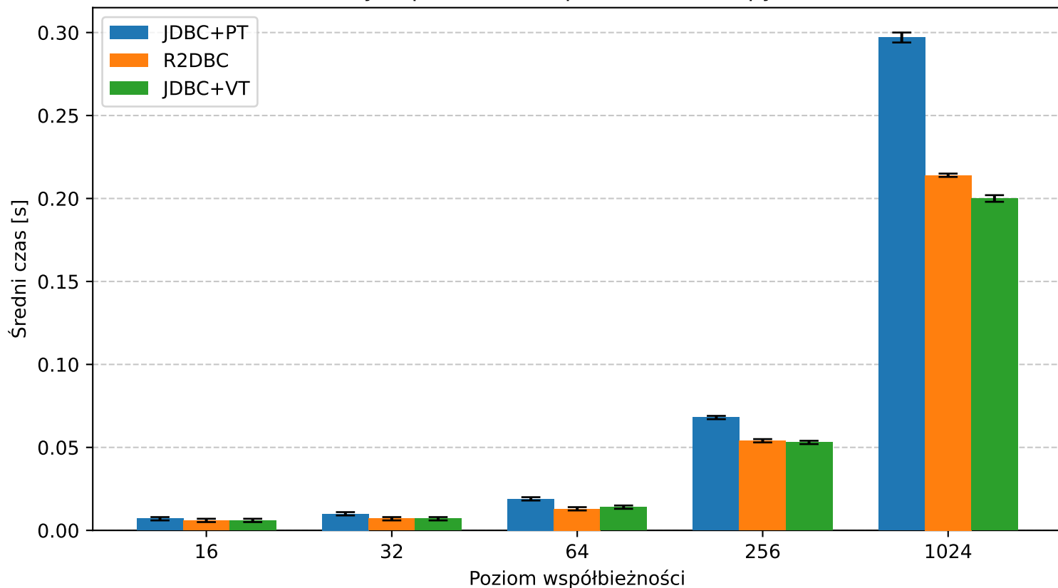
Porównanie średniego czasu trwania operacji dla różnych poziomów współbieżności (zapytanie Q2)
