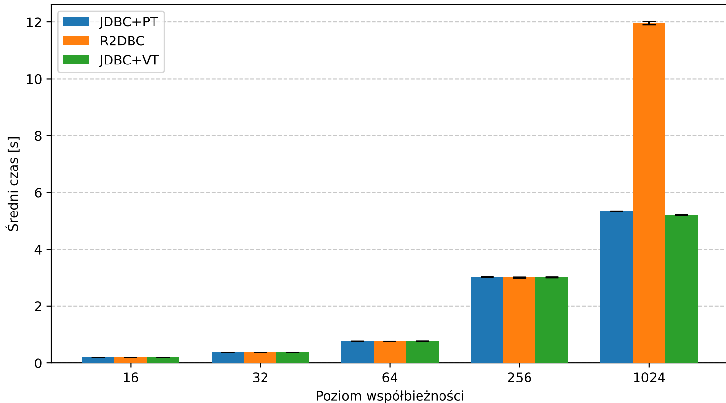
Porównanie średniego czasu trwania operacji dla różnych poziomów współbieżności (zapytanie Q3)
