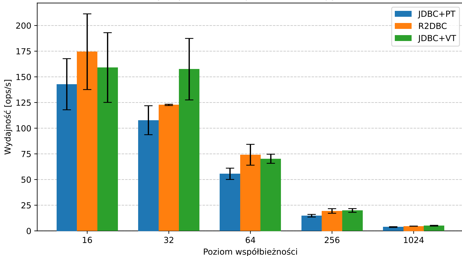
Porównanie wydajności scenariuszy dla różnych poziomów współbieżności (zapytanie Q2)
