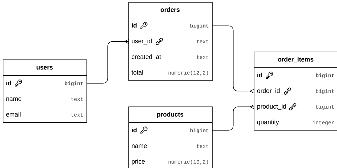
Rysunek 5.1: Schemat bazy danych wykorzystanej w ramach scenariusza \mathcal{A}
