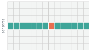
Atención temporal
