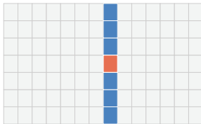
Atención espacial
