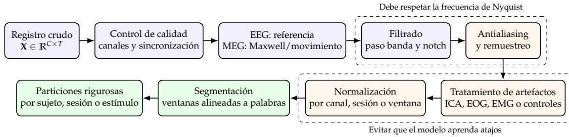
Figura 2.4: Flujo habitual de preparación de registros EEG y MEG para aprendizaje automático. El orden exacto puede variar, pero el filtrado antialiasing debe preceder al remuestreo y las particiones deben impedir fugas entre datos relacionados.
