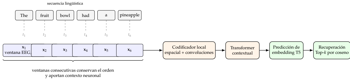
Figura 2.5: Esquema de clasificación contextual de palabras. Cada evento lingüístico define una ventana cerebral; las representaciones locales se contextualizan y se proyectan al espacio de un modelo de lenguaje para recuperar las palabras más próximas.
