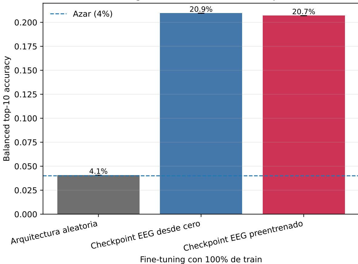
MEG-XL Figura 6 · vocabulario de 250 palabras
