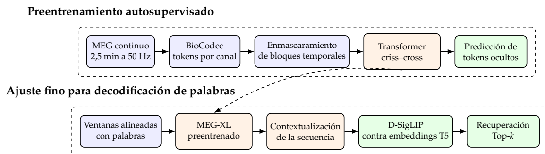
Figura 2.9: Resumen del preentrenamiento y del ajuste fino de MEG-XL. El modelo aprende primero a reconstruir tokens cerebrales en contextos largos y posteriormente reutiliza esas representaciones en una tarea contrastiva de clasificación contextual de palabras. Adaptado conceptualmente de Jayalath y Parker Jones.
