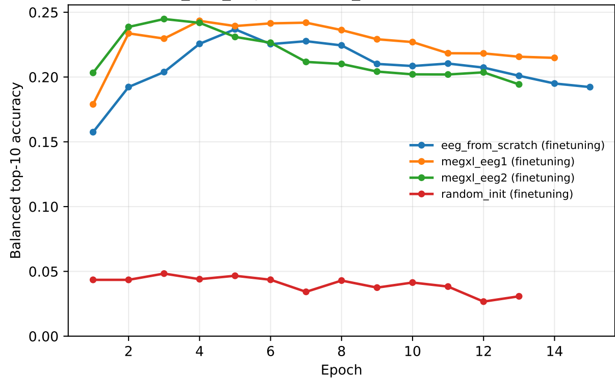
ds004408_four_way 20260703_120008 · val · retrieval 250
