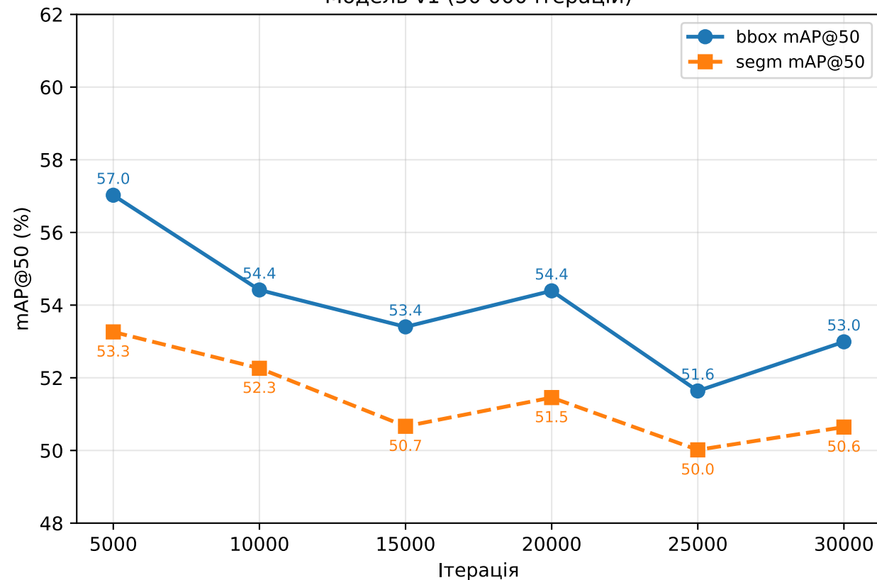
Модель v1 (30 000 ітерацій)
