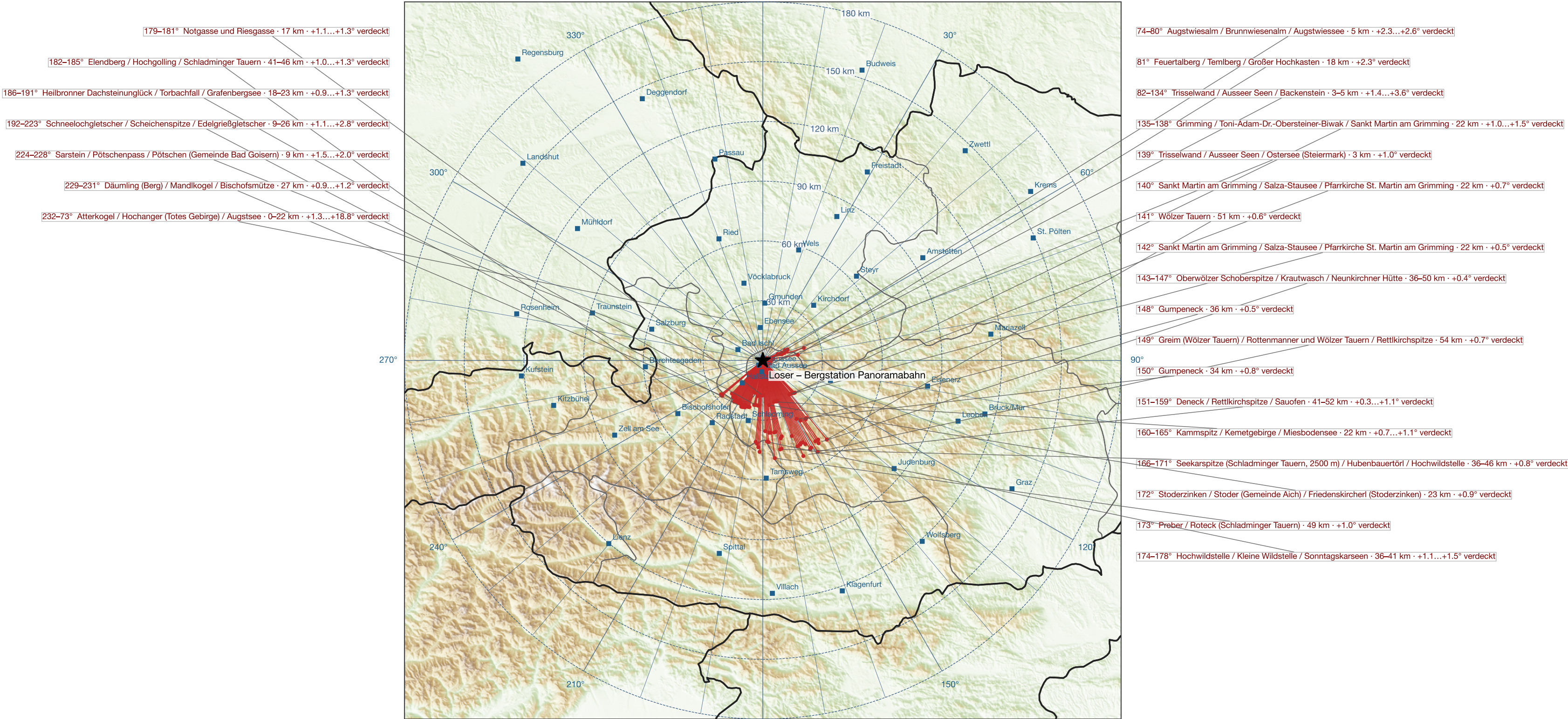
Loser – Bergstation Panoramabahn – Zoom 180 km, 360°: das Gelände, das in jeder Richtung den Horizont bildet (Peilung · Name · Entfernung · Winkel zur Waagrechten) grün = frei (unter der Waagrechten), orange = knapp (–0,3...0°), rot = Terrain über der Waagrechten · Relief SRTM1 · Staatsgrenzen dick, Bundesländer dünn · 10 m Antenne, 4/3-Erde
