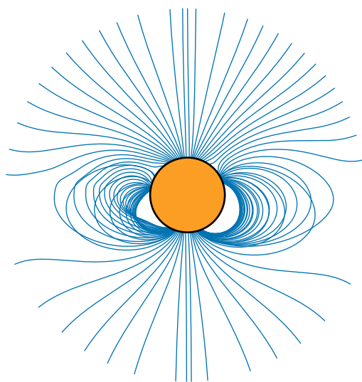
PFSS, r_{ss} = 5.0R_{\odot}
