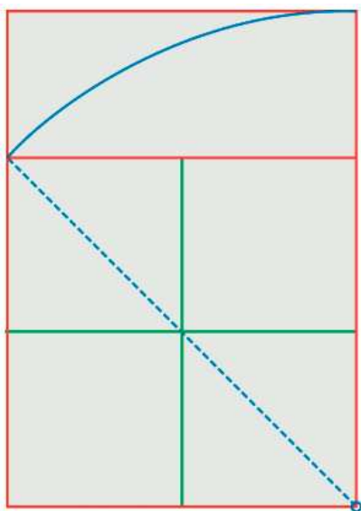
Figura 3a. Schema proporzionamento della lastra col rettangolo \sqrt{2} attraverso il ribaltamento della diagonale del quadrato costruito sul lato corto.
