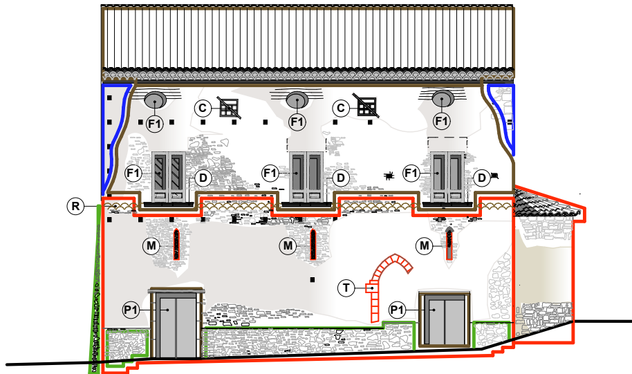
PROSPETTO SUD
