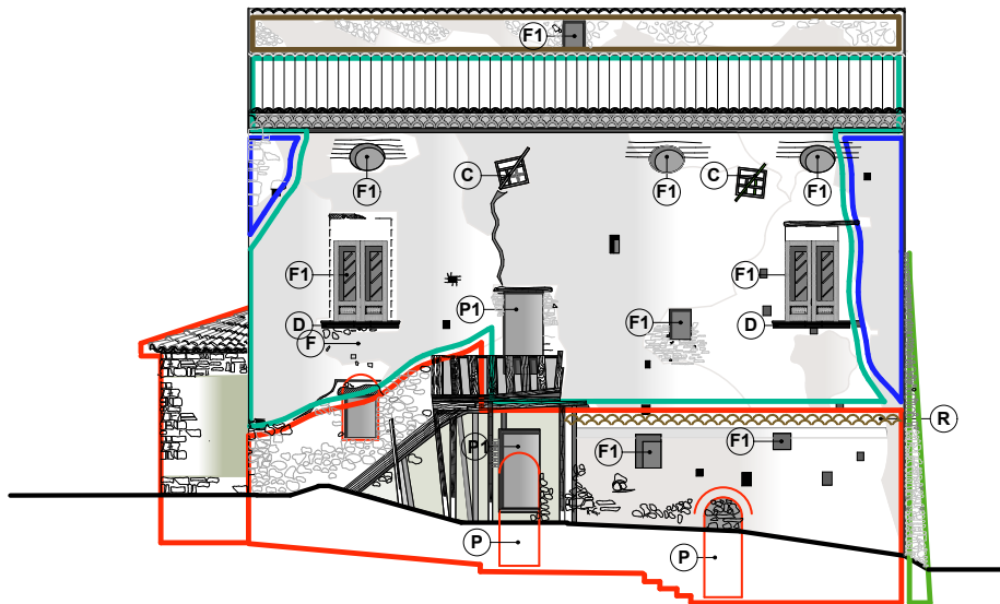
PROSPETTO NORD
