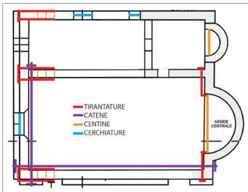
fig. 170 - Pianta dell'edificio con indicazione dei punti di inserimento dei presidi antisismici, tiranti, catene, centine (dis. P. Lopetrone).
