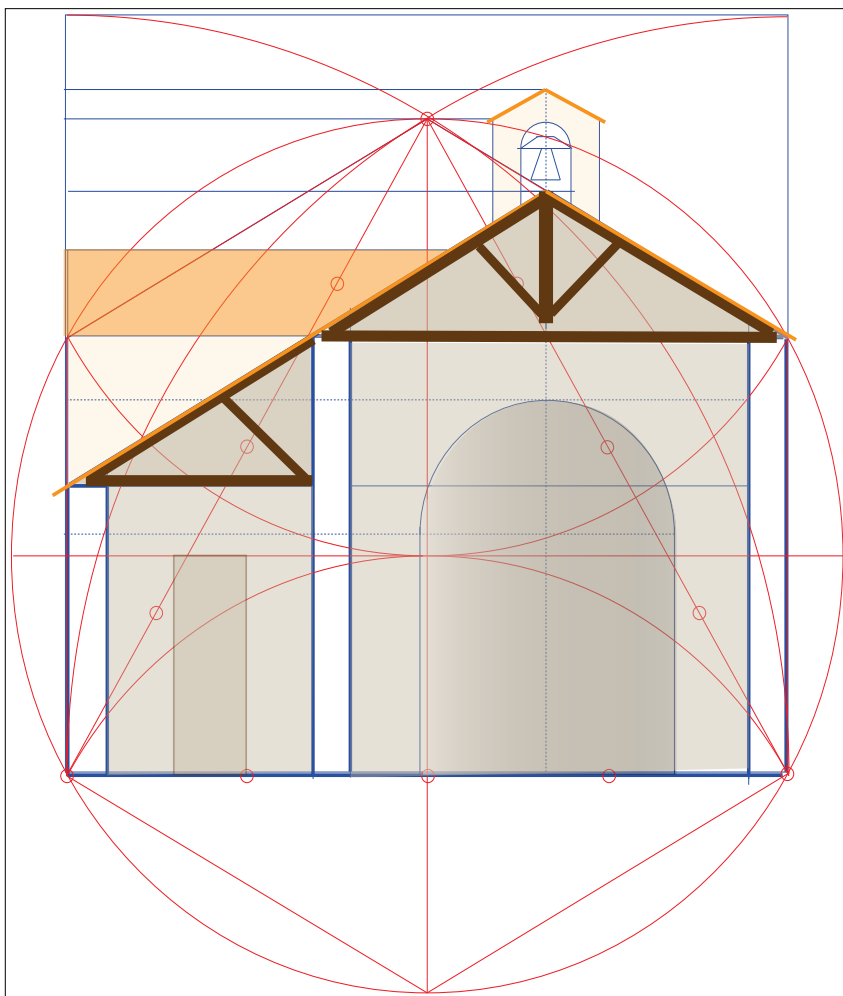
fig. 73 - Proporzionamento delle altezze della chiesa sulla sezione trasversale attraverso l'esagramma, (dis. P. Lopetrone).
