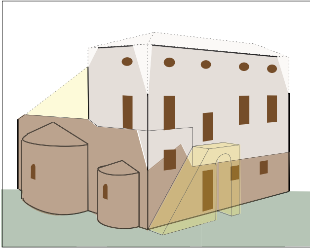
fig. 108 - Danni provocati dal sisma del 1783, (dis. P. Lopetrone).
