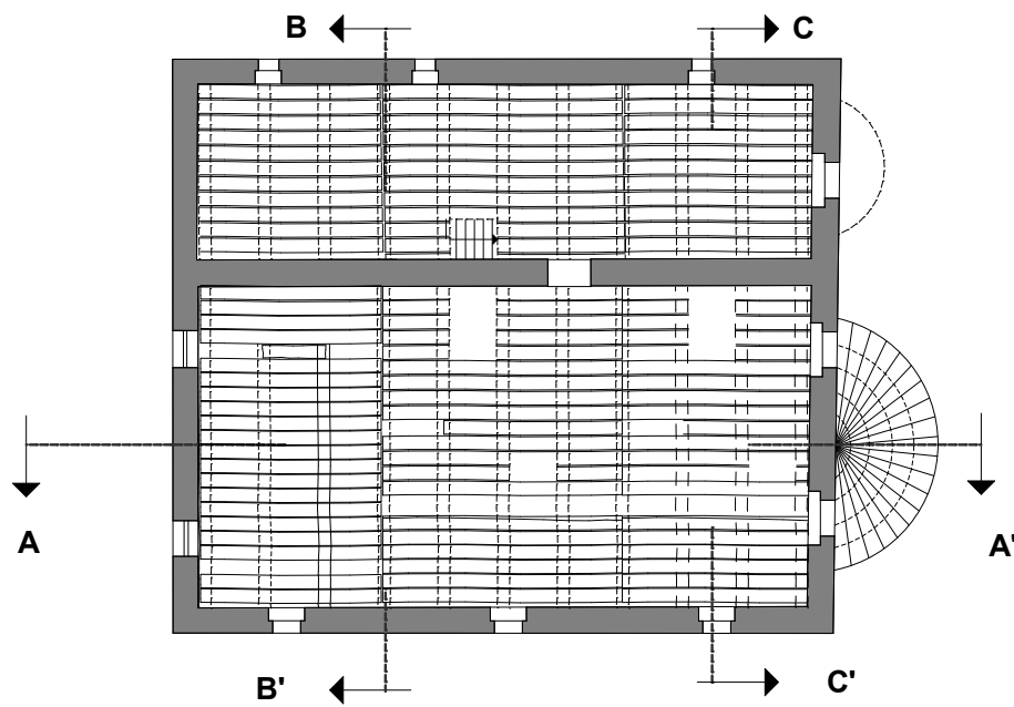
PIANTA PIANO SOTTOTETTO RILIEVO
