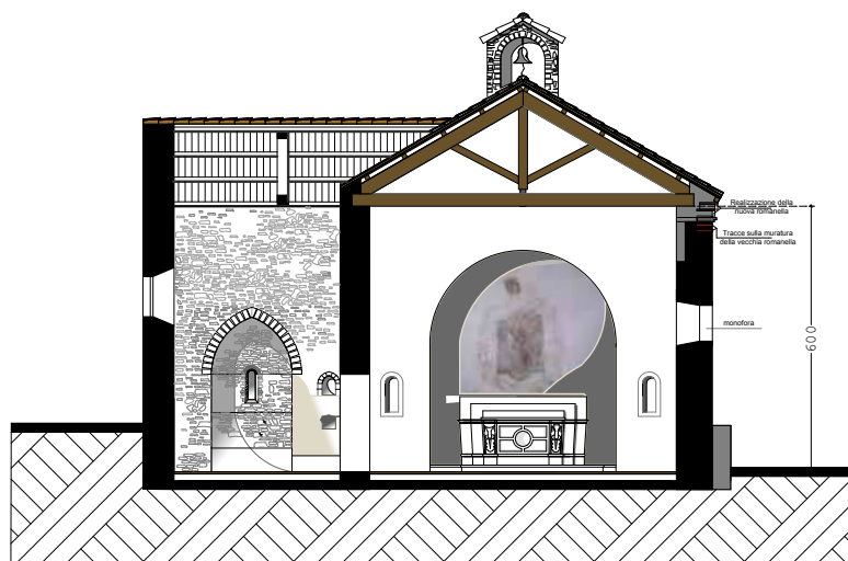
SEZIONE STATO FUTURO C - C'
