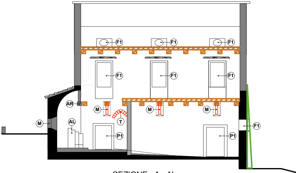
SEZIONE A - A'
