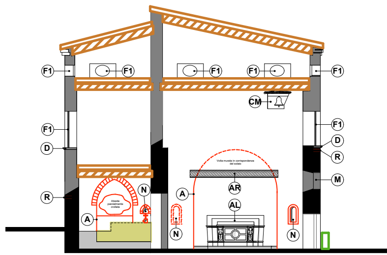
SEZIONE C - C'
