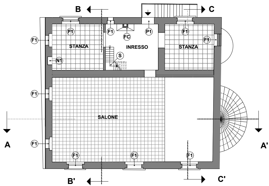
PIANTA PIANO PRIMO RILIEVO
