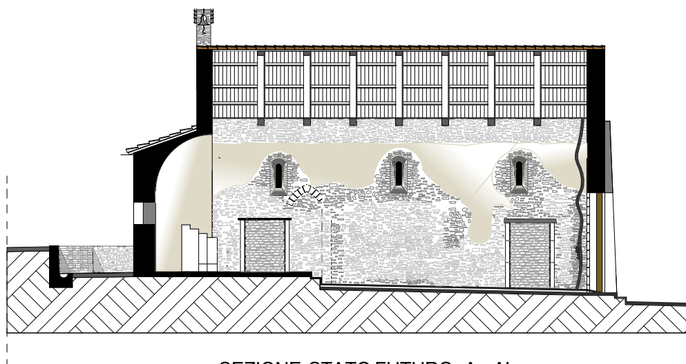
SEZIONE STATO FUTURO A - A'
