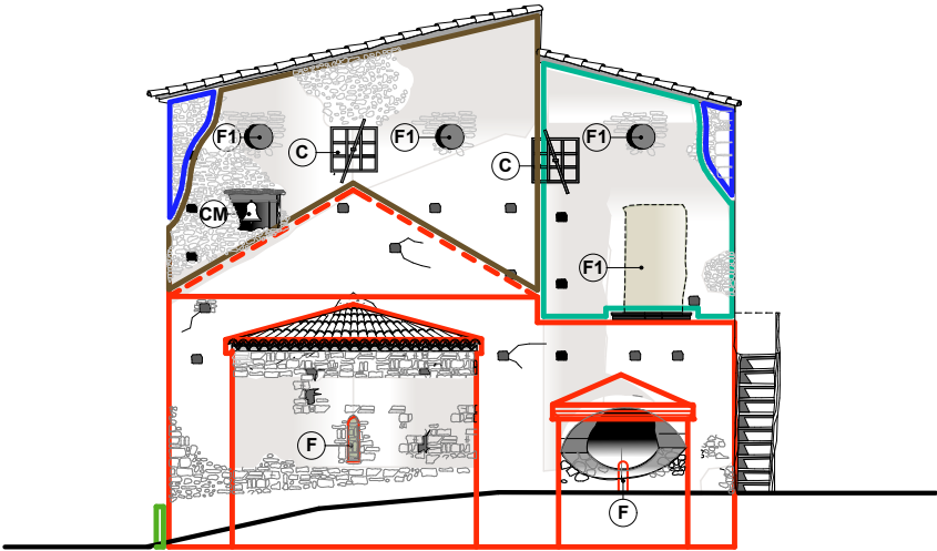
PROSPETTO EST
