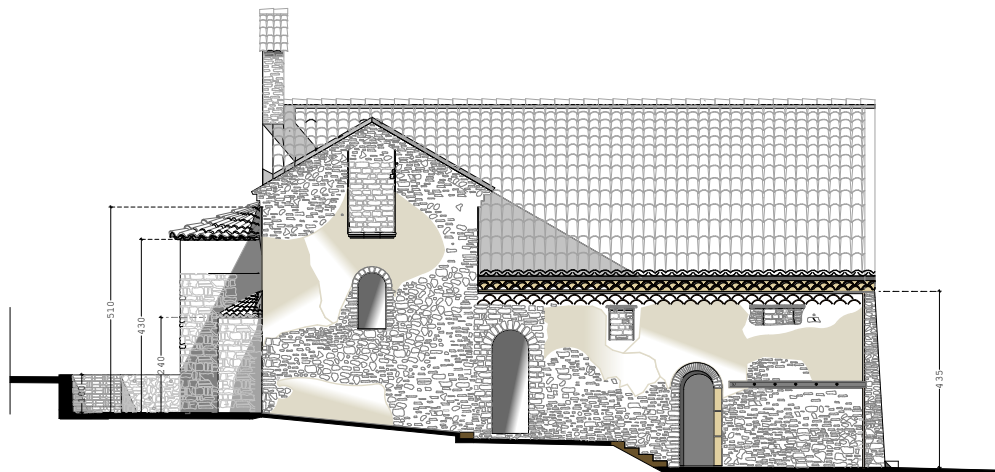
PROSPETTO NORD
