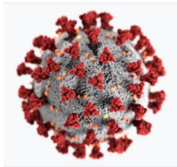
Gambar 1. Ilustrasi Morfologi dari Coronavirus
