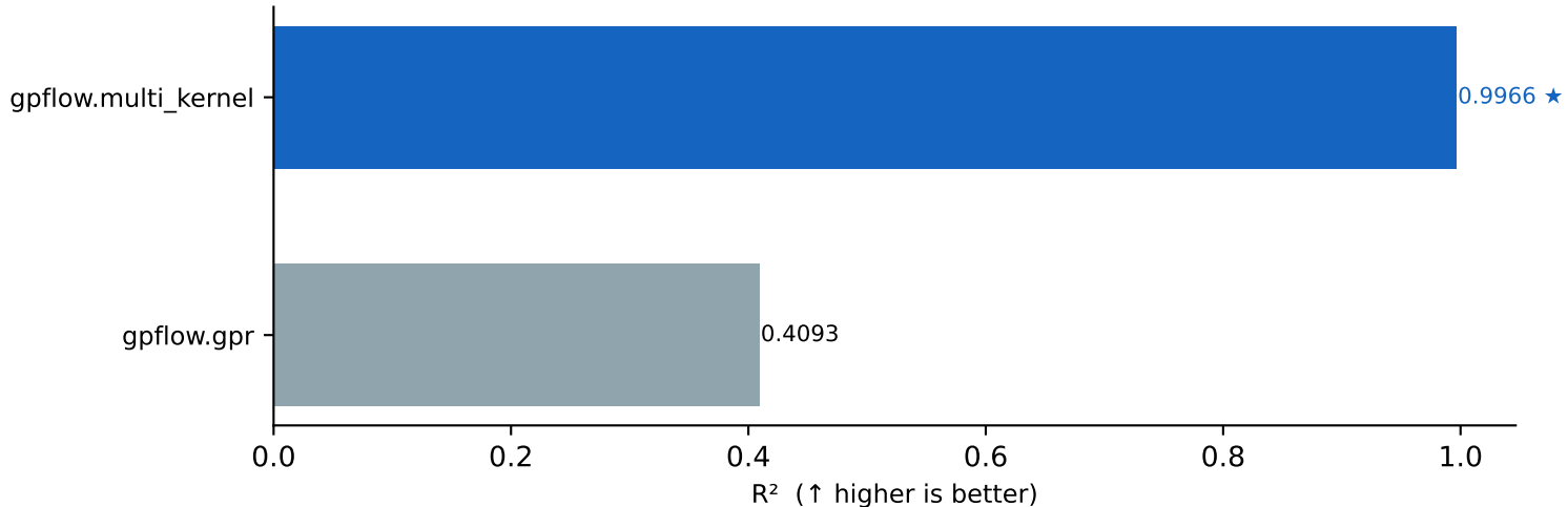
tabular.energy_efficiency — R^2
