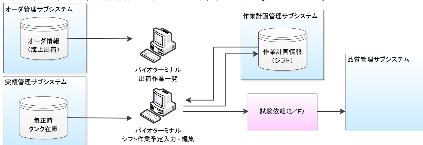
図 3. 2. 3. -1 シフト作業計画情報登録の機能相関図
