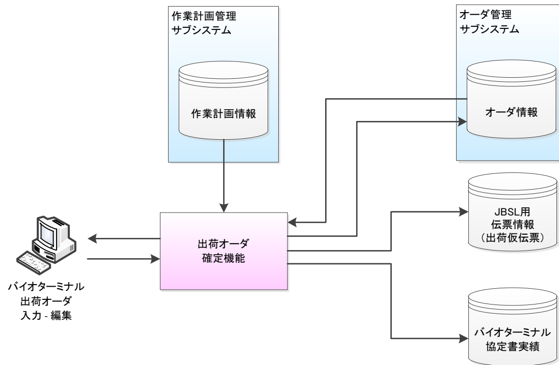
図 3.1.2. -5 出荷オーダー確定の機能相関図
