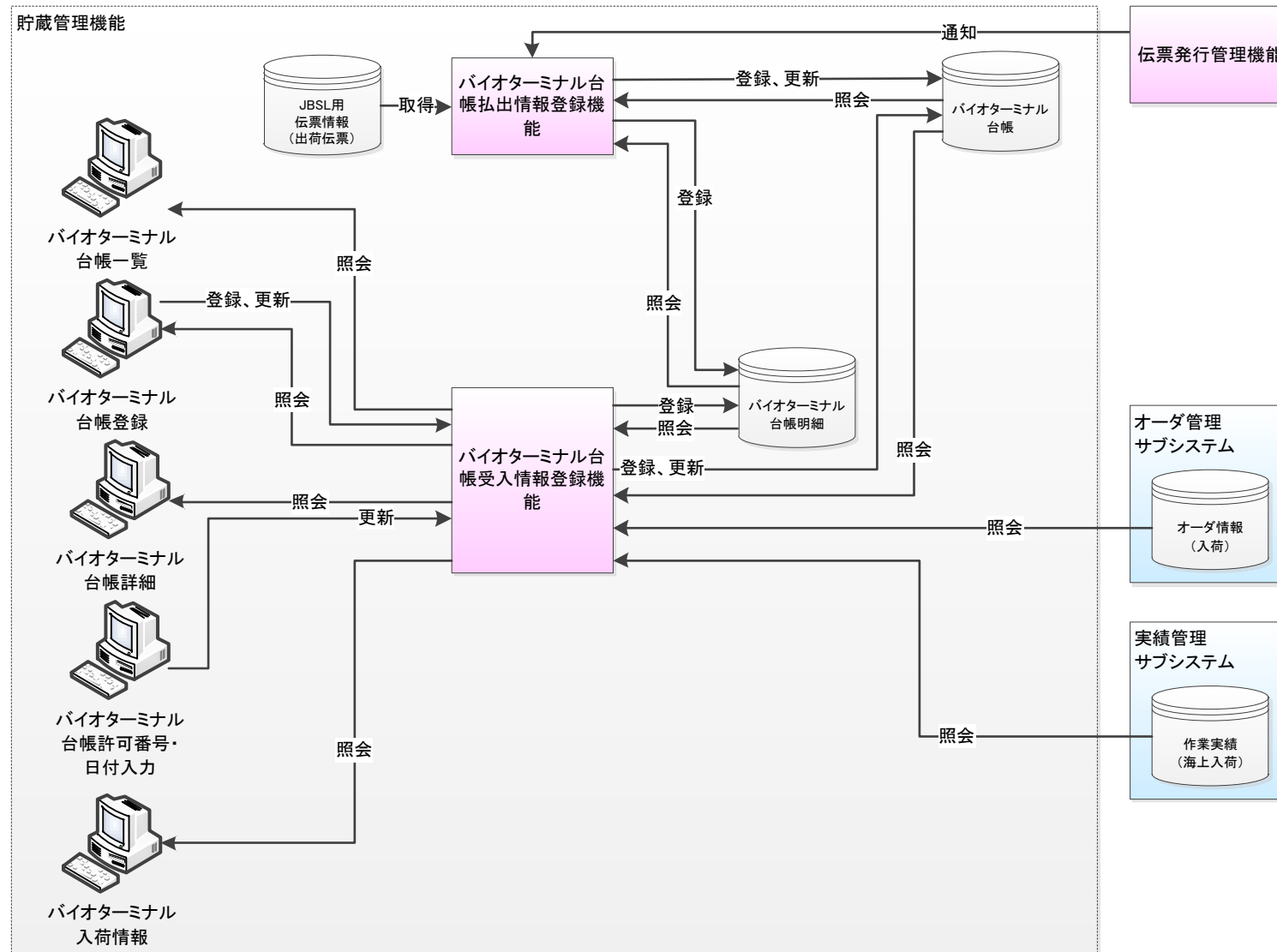
図 3.6.-1 貯蔵管理機能の機能相関図
