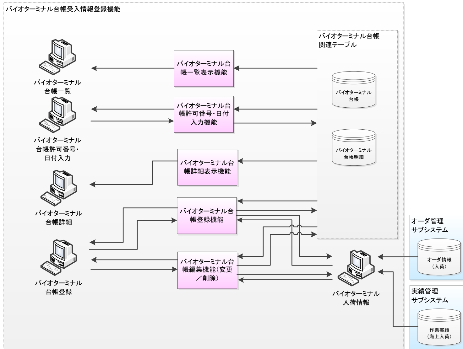
図 3.6.1.-1 バイオターミナル台帳受入情報登録機能の機能相関図
