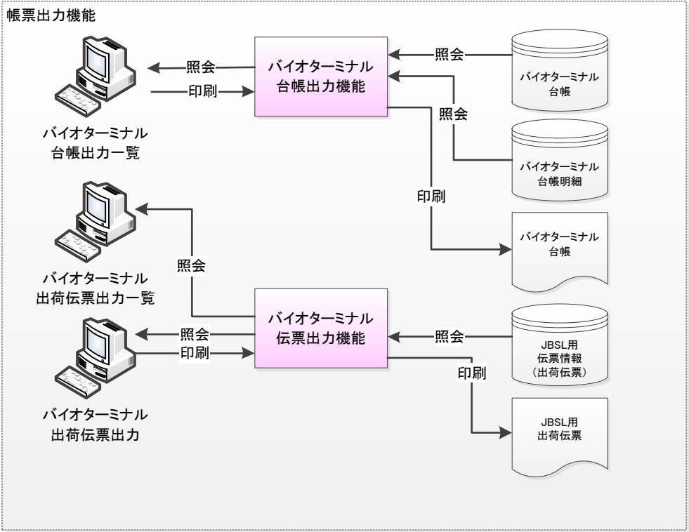
図 3. 7. -1 帳票出力機能の機能相関図
