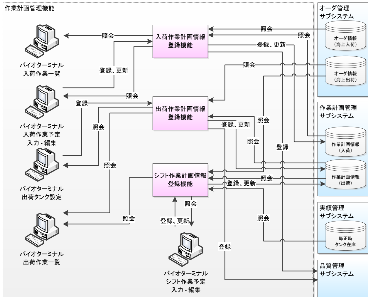
図 3. 2. -1 作業計画管理機能の機能相関図
