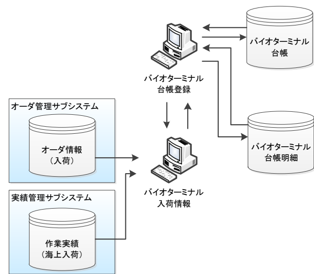
図 3. 6. 1. -4 バイオターミナル台帳登録機能の機能相関図
