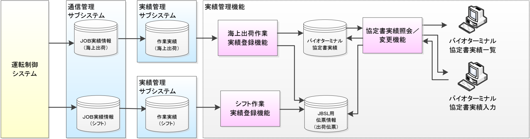
図 3. 4. -1 実績管理機能の機能相関図
