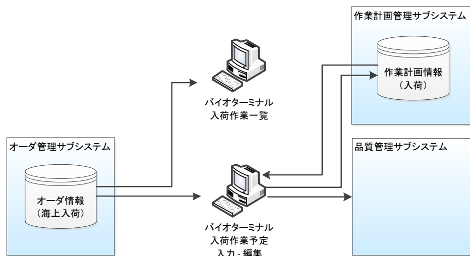
図 3.2.1.-1 入荷作業計画情報登録の機能相関図
