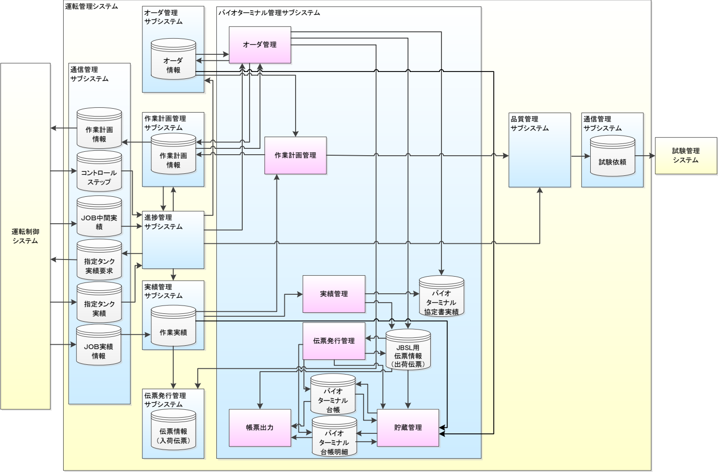
図 1.2.-1 バイオターミナル管理サブシステムの機能相関図
