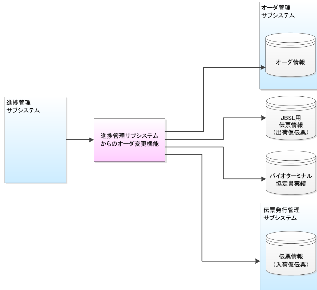
図 3.1.2.-7 進捗管理サブシステムからのオーダー変更機能の機能相関図
