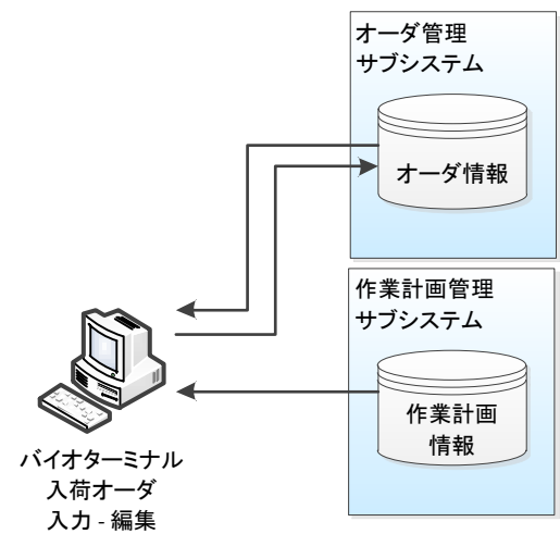
図 3. 1. 1. -5 オーダー確定の機能相関図
