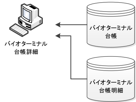
図 3.6.1.-13 バイオターミナル台帳詳細表示機能の機能相関図
