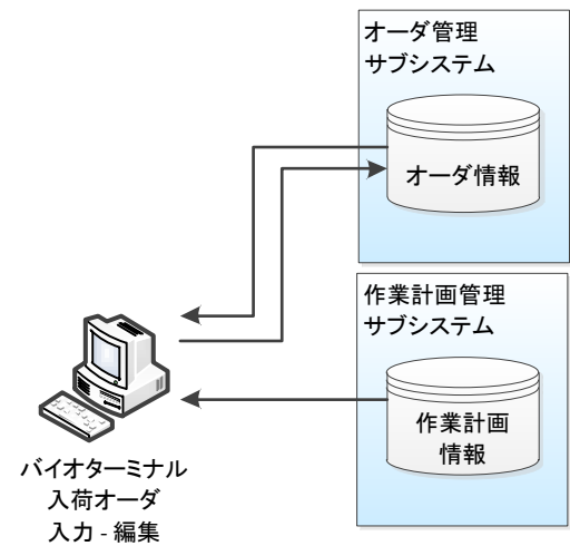
図 3. 1. 1. -3 入荷オーダー追加／変更／削除の機能相関図
