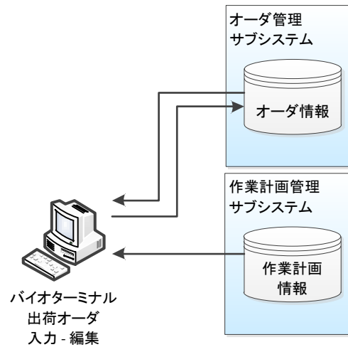
図 3.1.2.-3 出荷オーダー追加／変更／削除の機能相関図
