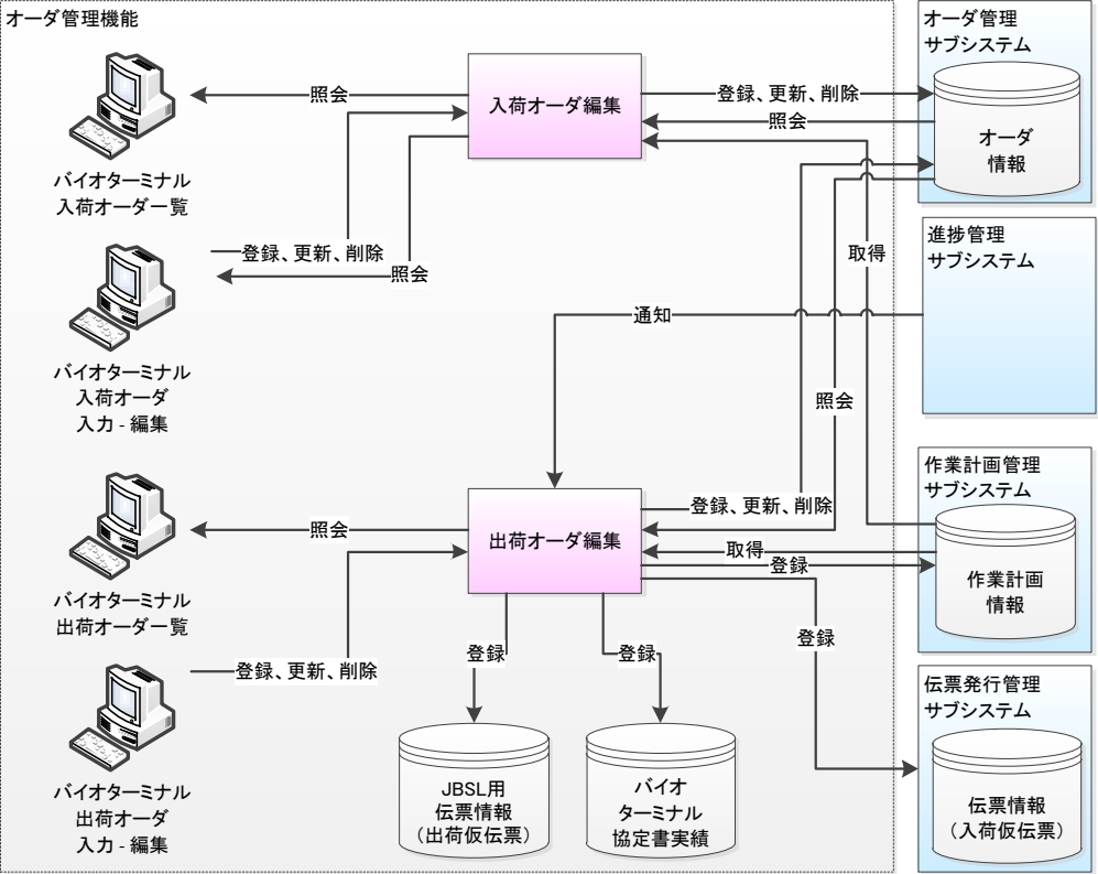
図 3.1.-1 オーダ管理機能の機能相関図
