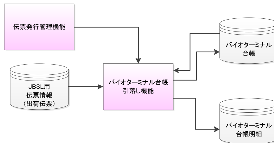
図 3.6.2.-1 バイオターミナル台帳引落とし機能の機能相関図
