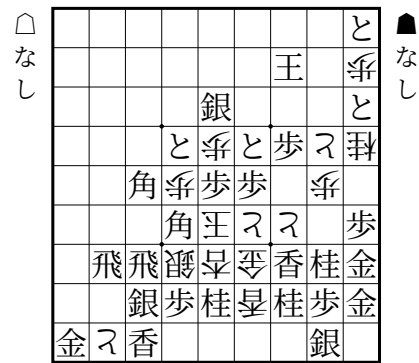
盤上 40 枚 → 盤上 3 枚（113 手の最短解は 1 通り）
