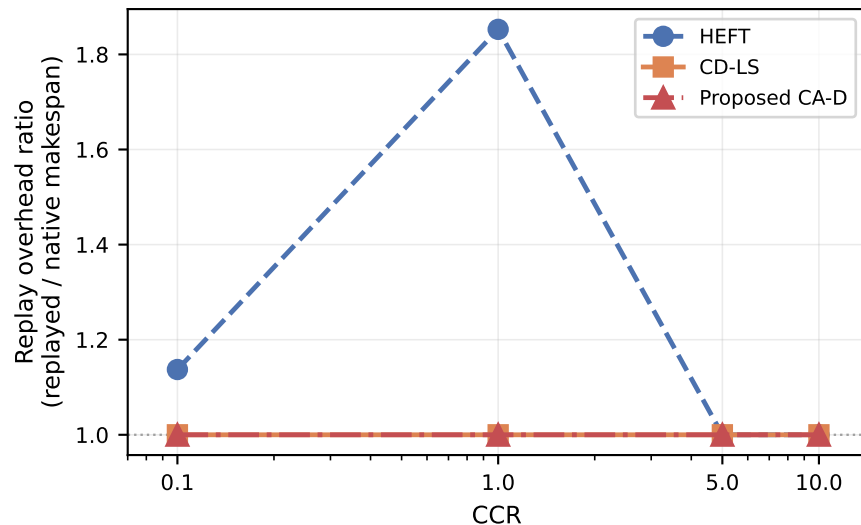
Fork-join
