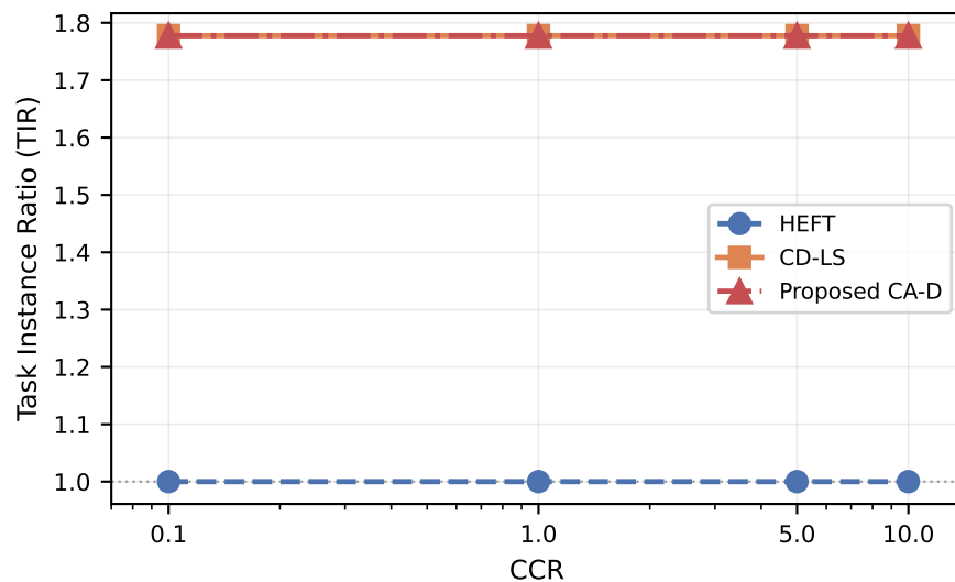
Fork-join
