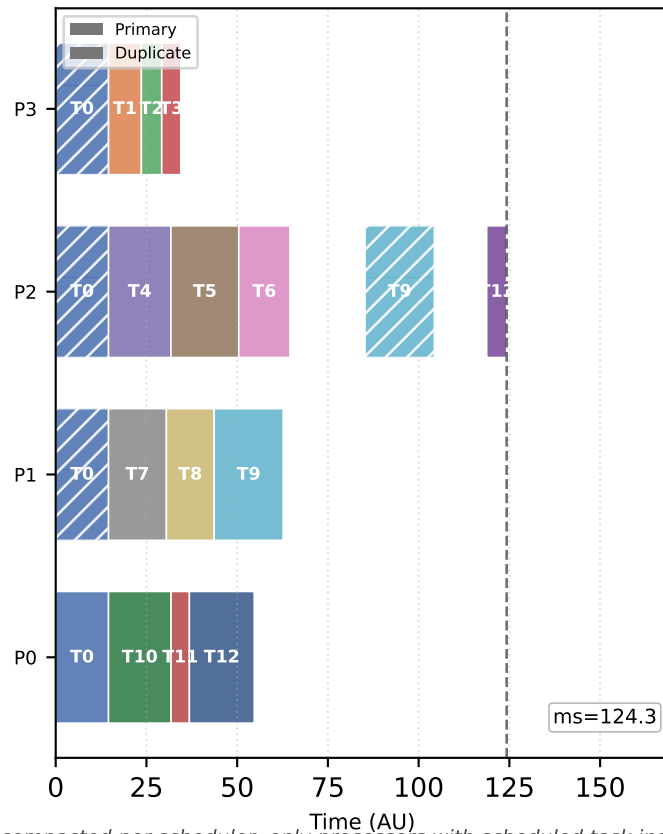
CD-LS
