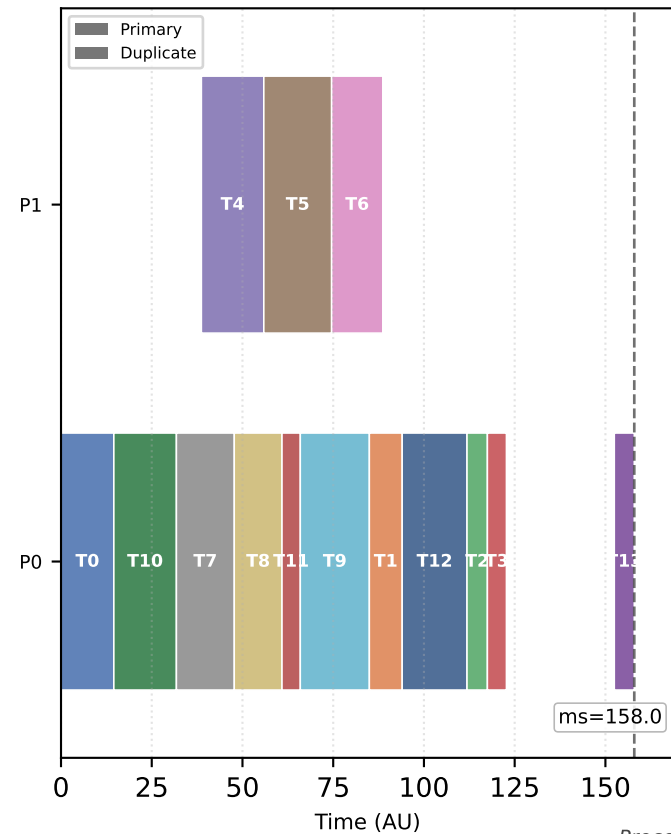
HEFT
